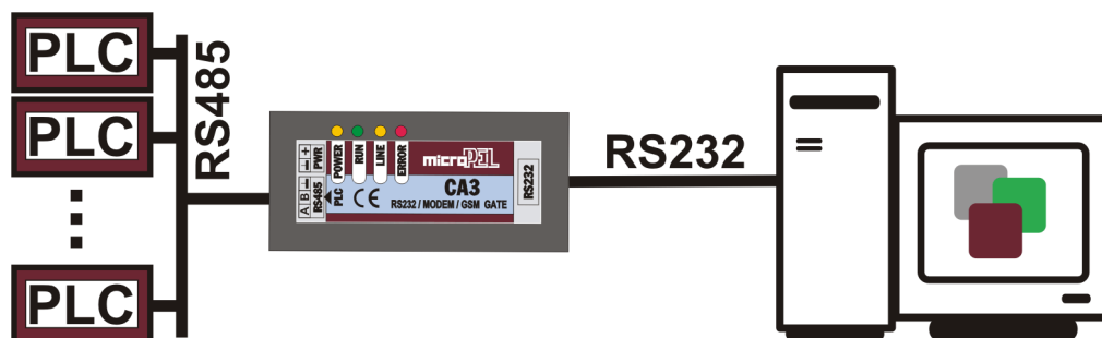
Obr. 1: Propojení CA3 s PC pomocí sériového kabelu
