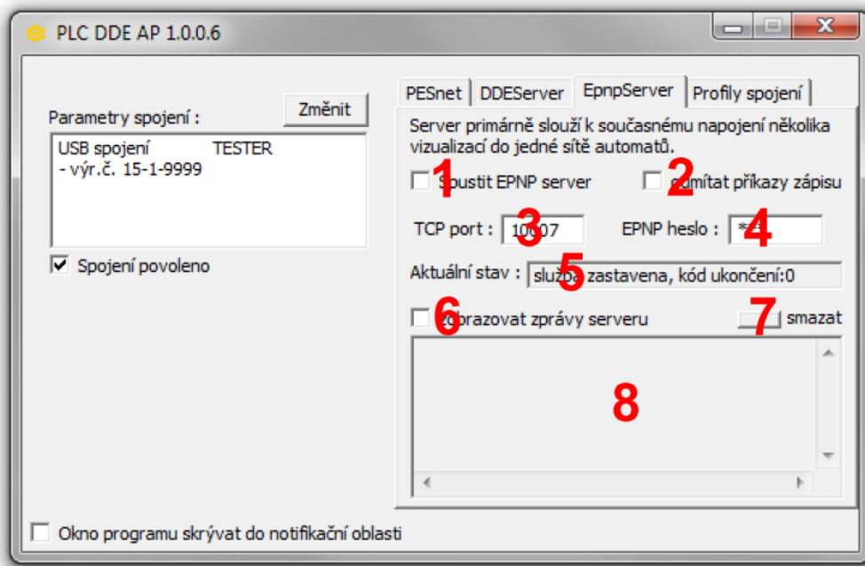
Obr. 4 - Okno programu DdeAP se zobrazenou kartou nastavení pro EPNP server
